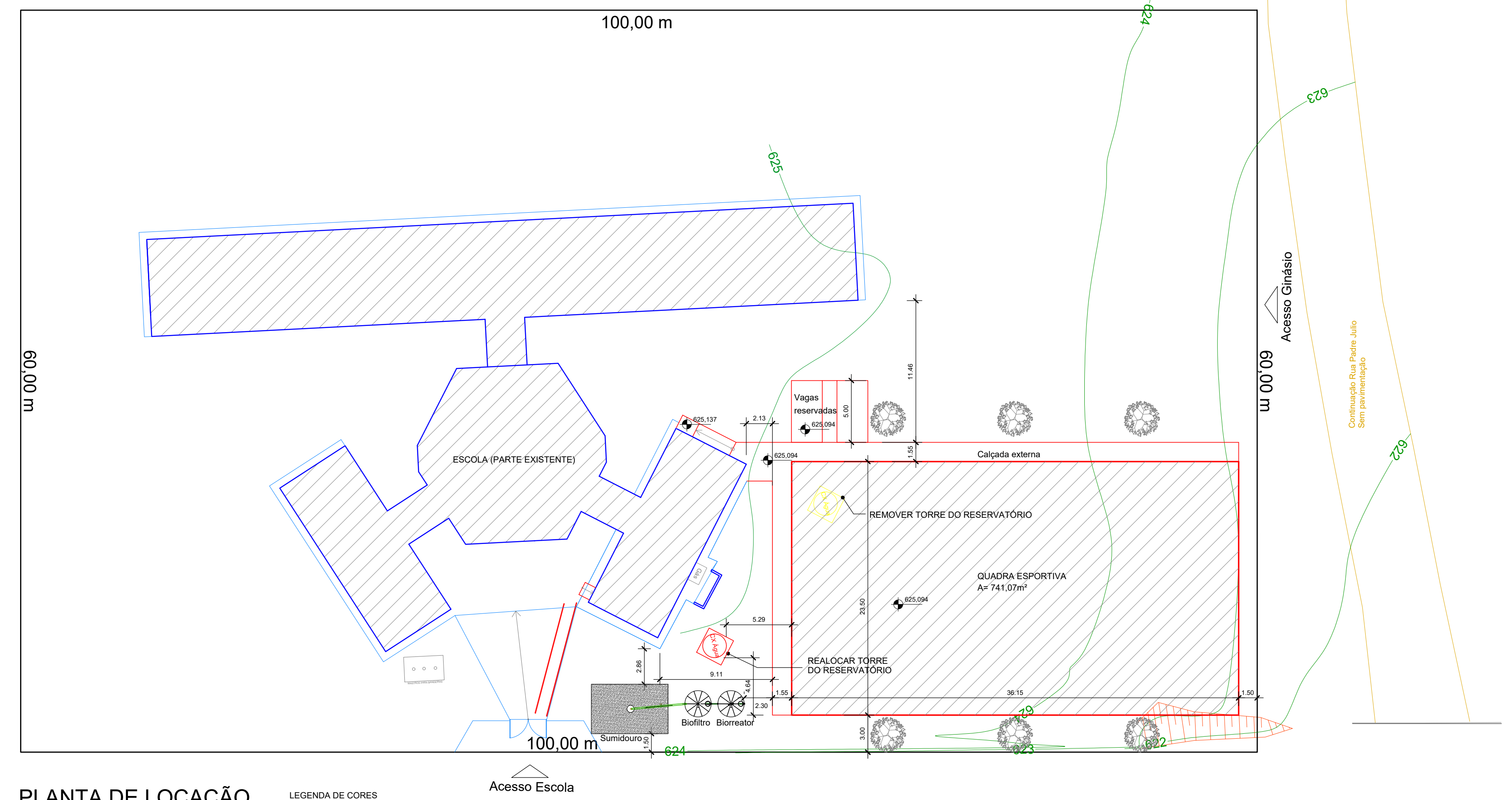
PLANTA DE LOCAÇÃO ESC: 1/250
