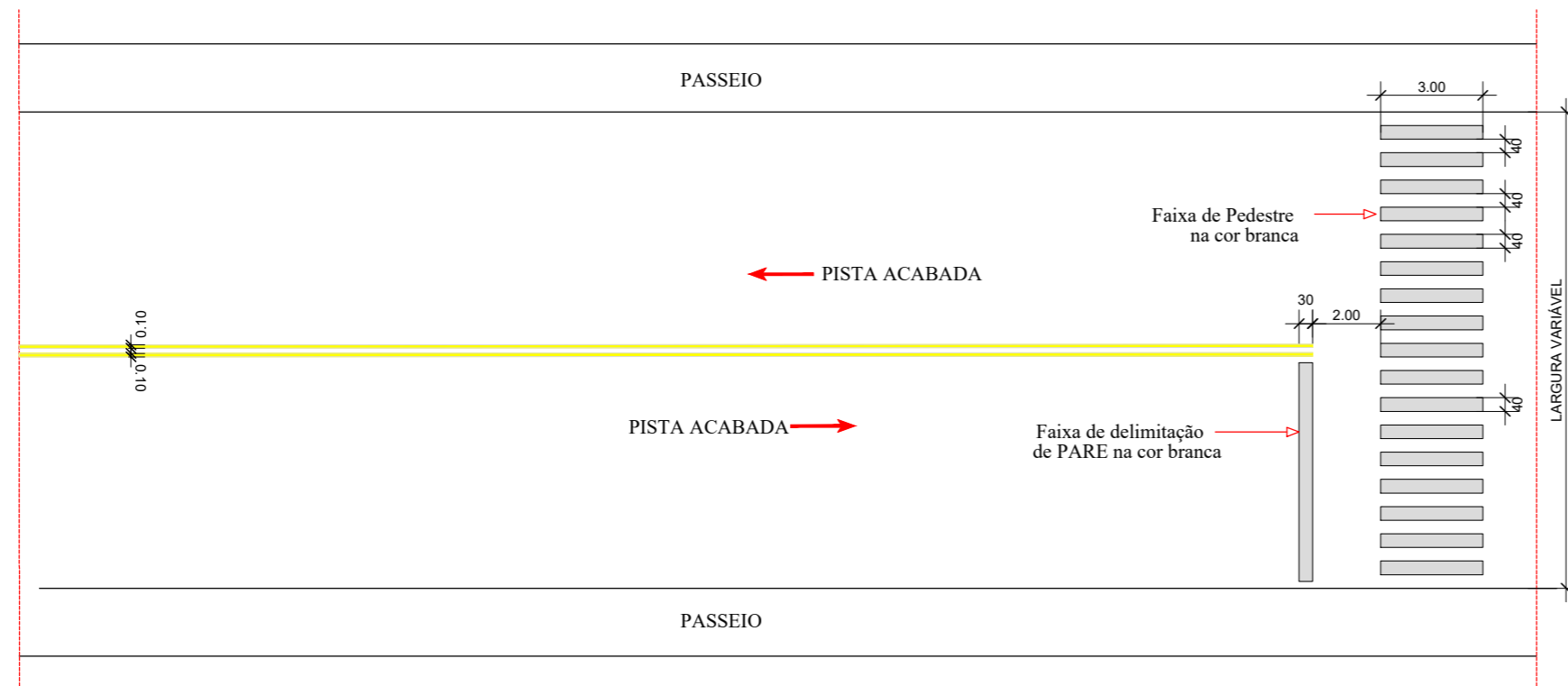
DETALHE DE SINALIZAÇÃO HORIZONTAL ESC.: 1:200
