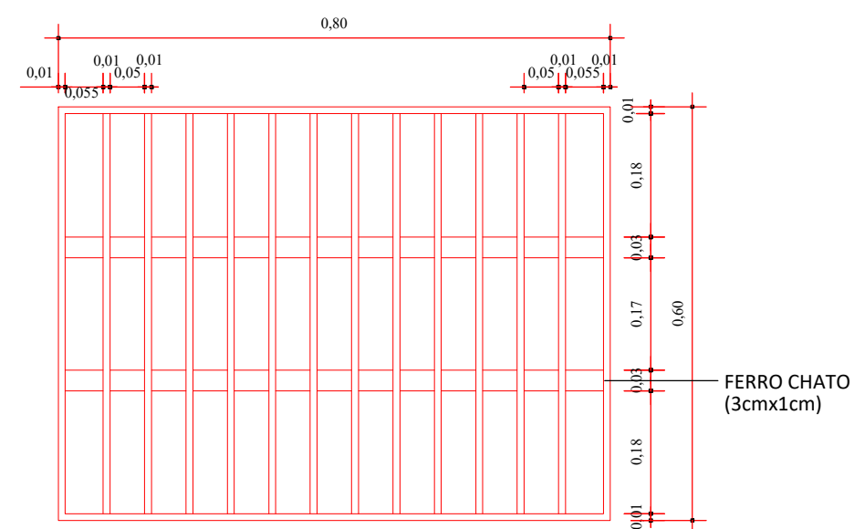
PLANTA - GRELHA
