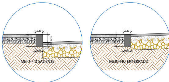
DETALHE 01
