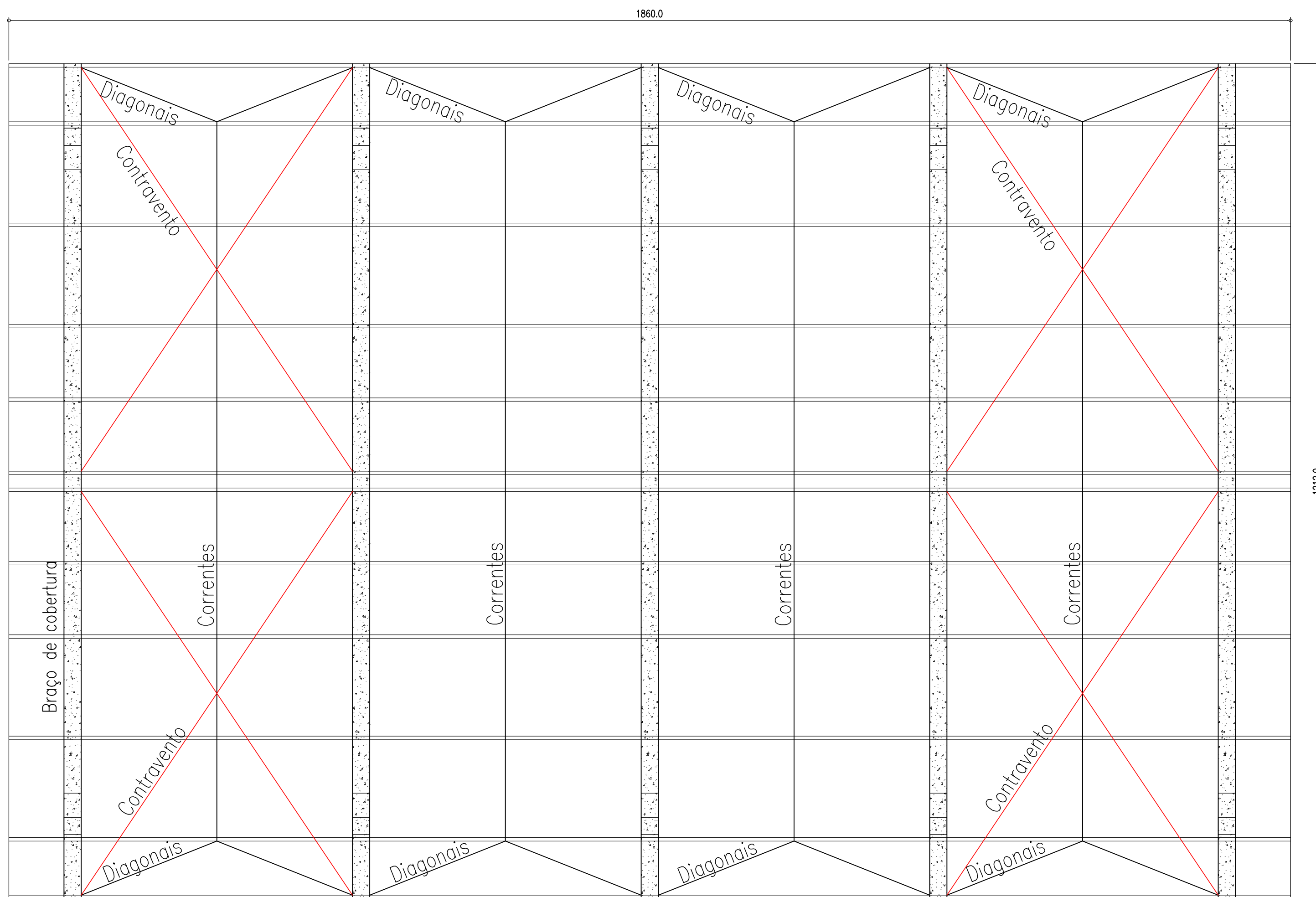
Detalhamento: Cobertura Escala: 1:50
