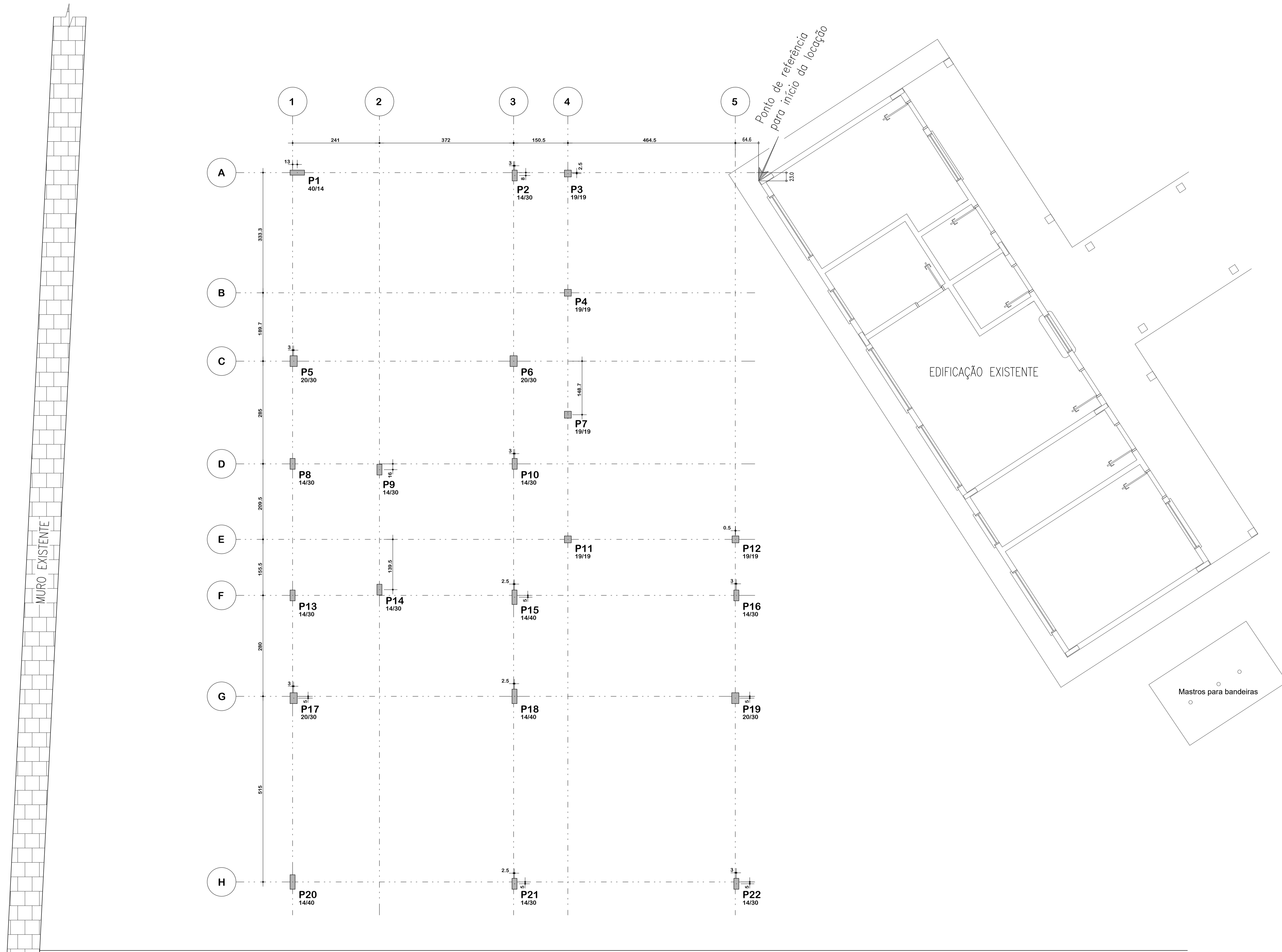
Planta Baixa: Locação dos pilares Escala: 1:50
