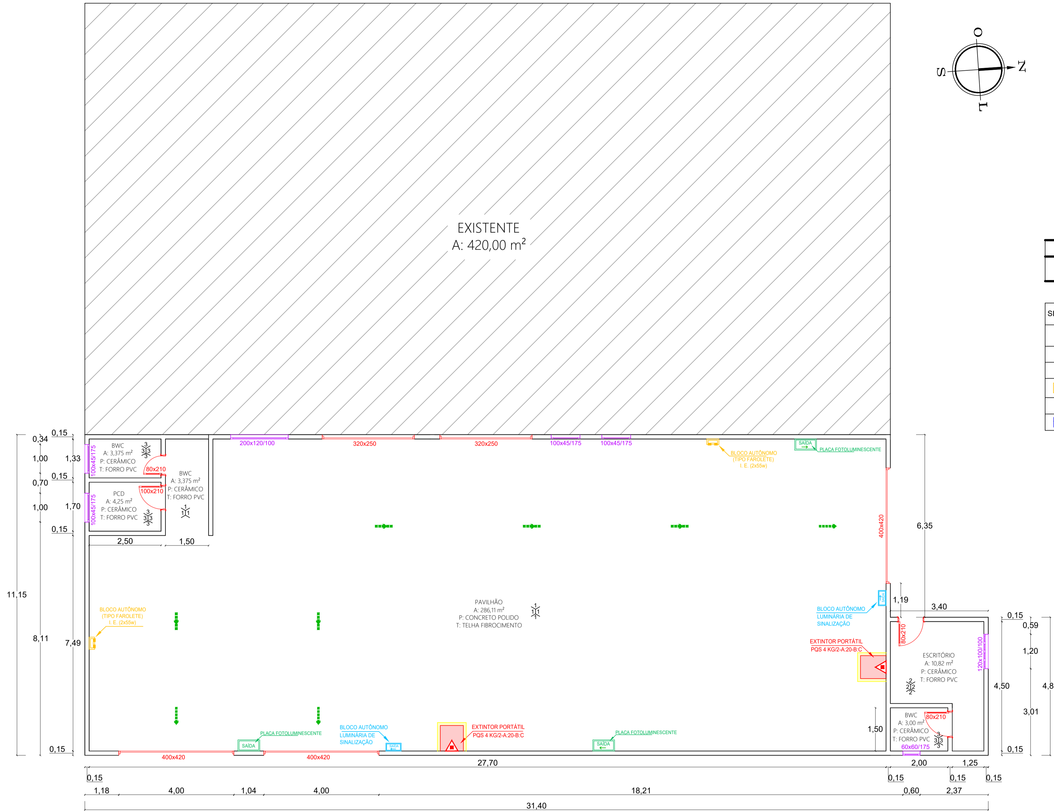
Planta Baixa - PPCI Escala 1:75
