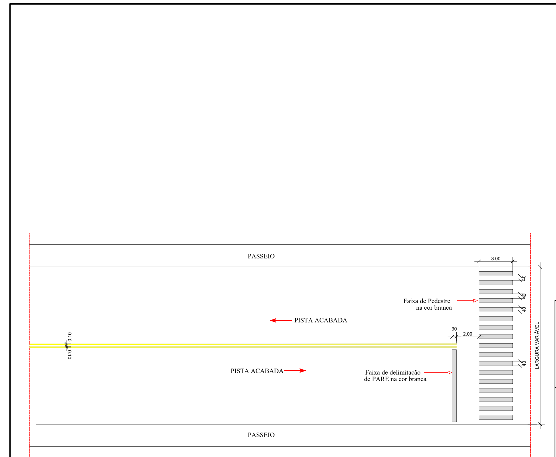
DETALHE DE SINALIZAÇÃO HORIZONTAL ESC.: 1:200
