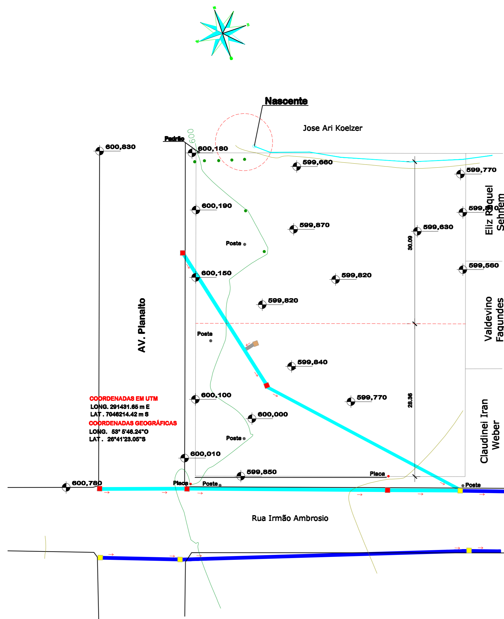
LEVANTAMENTO PLANIALTIMÉTRICO ESC.: 1/500
