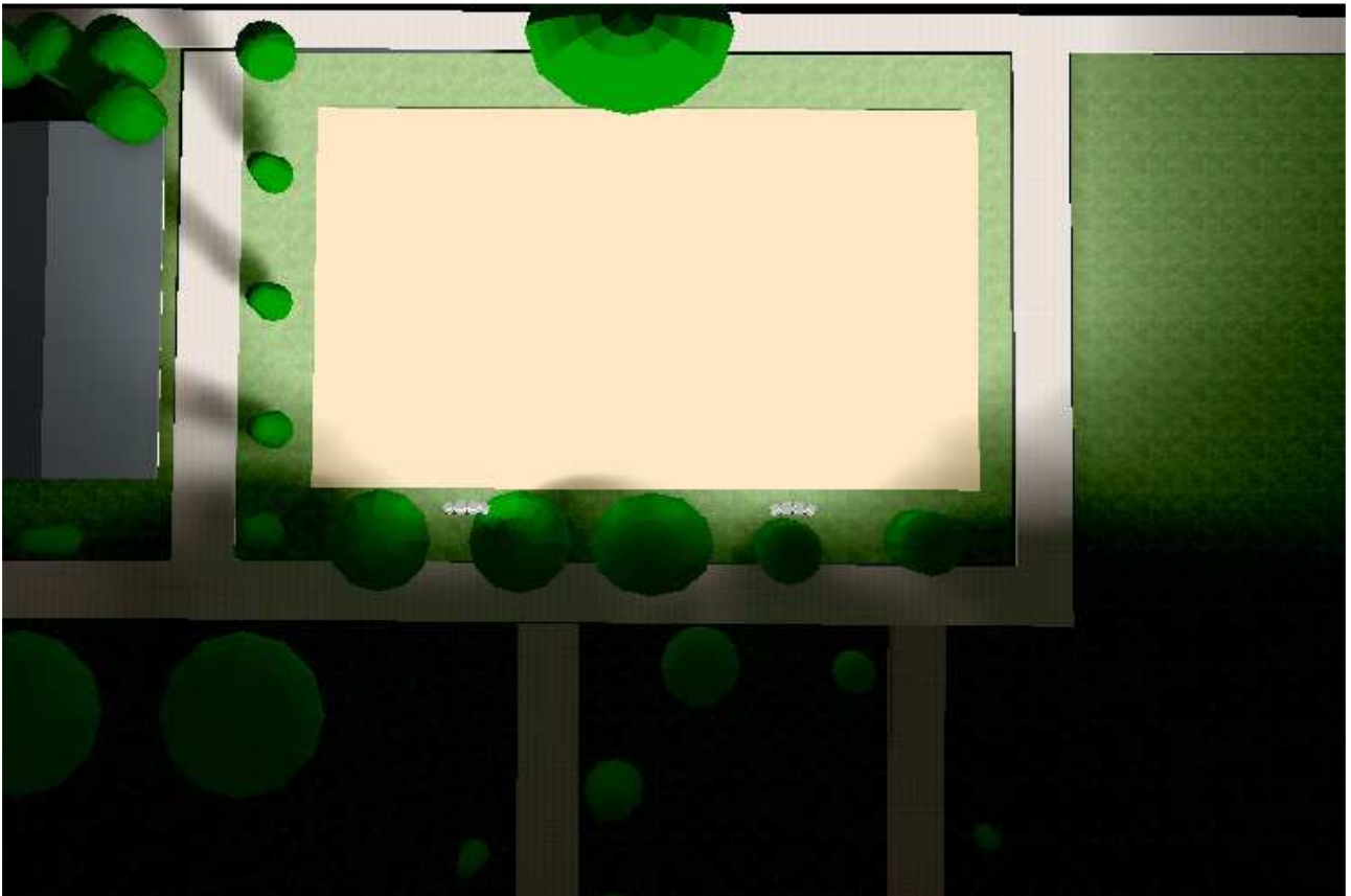
Simulação da iluminação da quadra de areia através do software Dialux.
